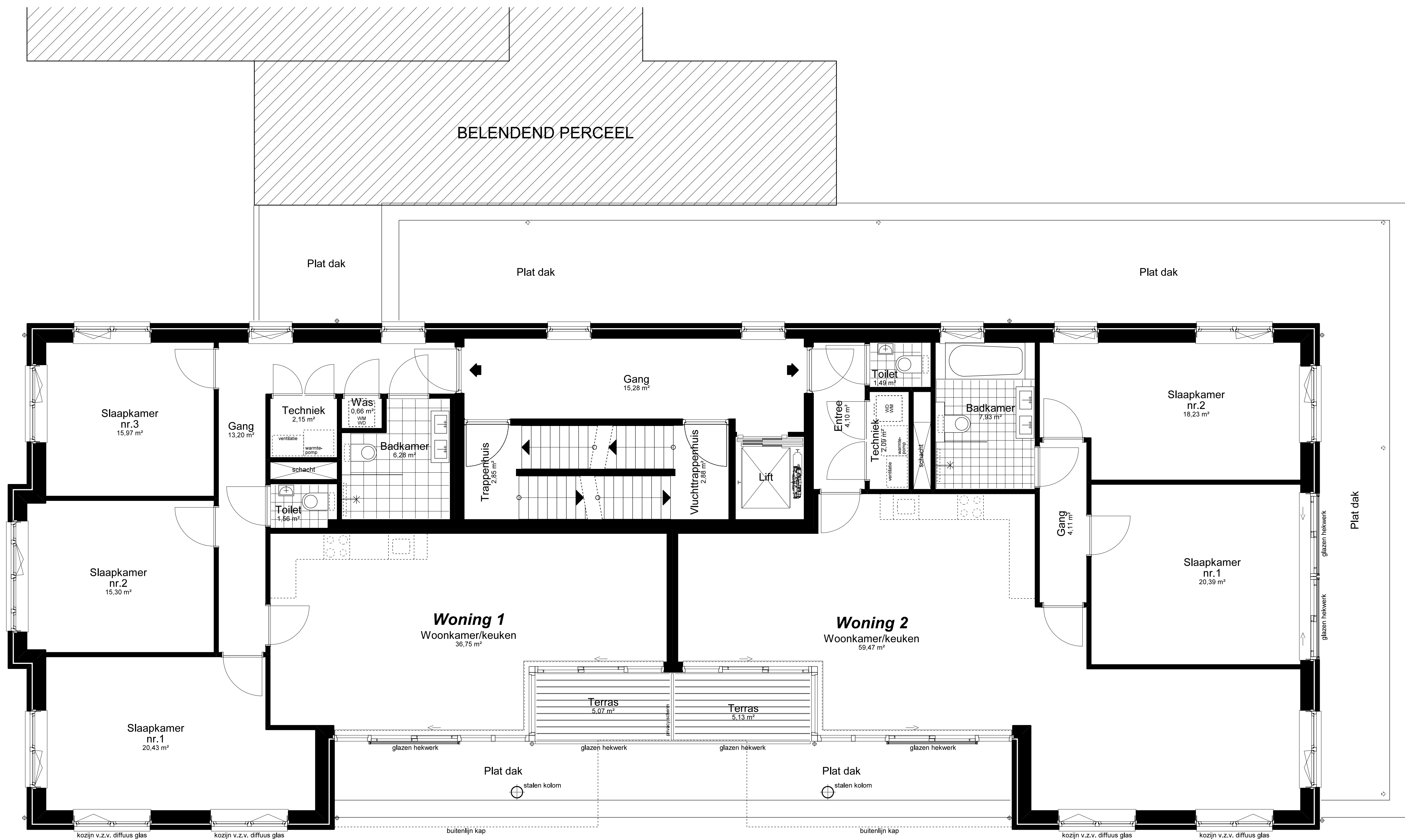
1e VERDIEPING
