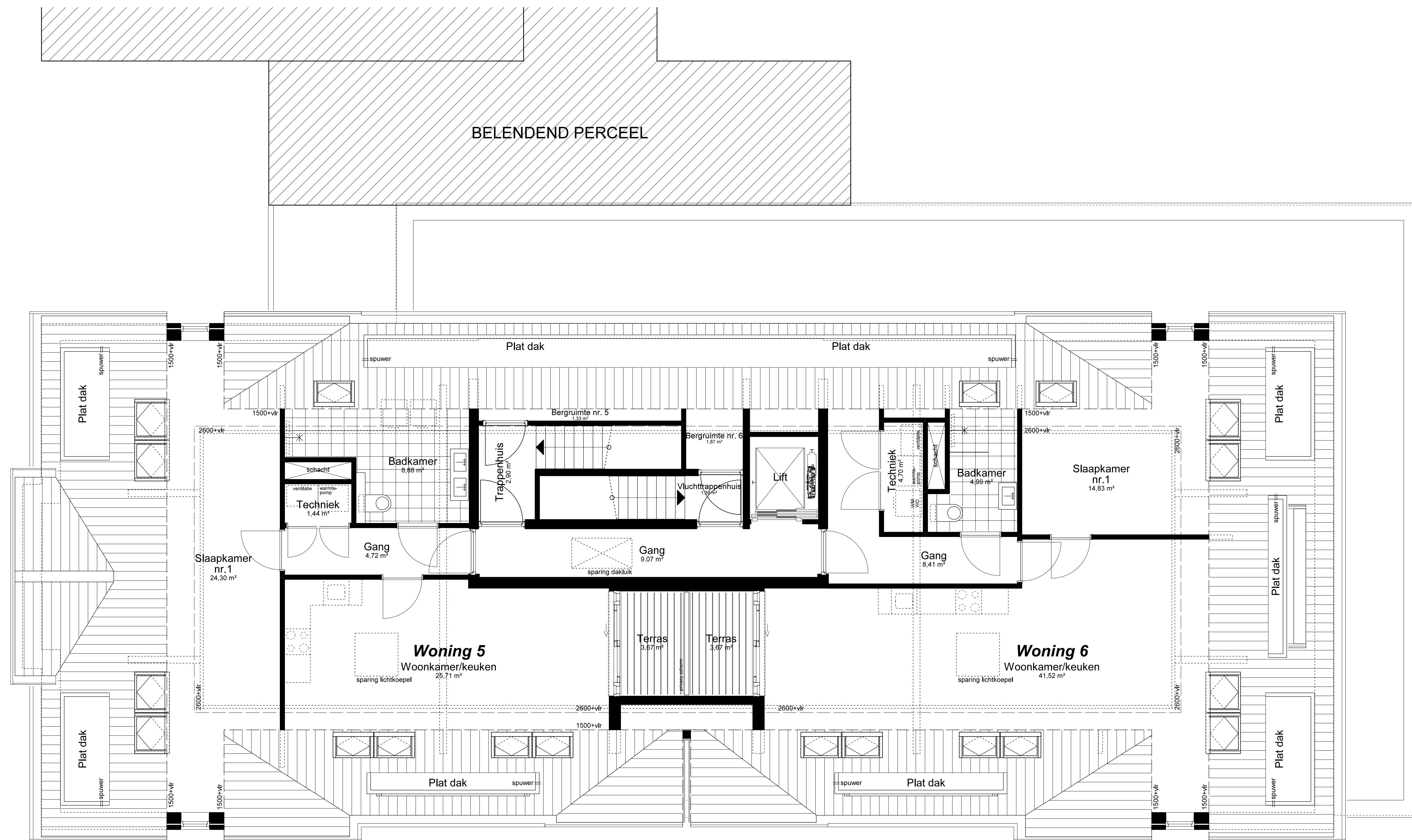
3e VERDIEPING
