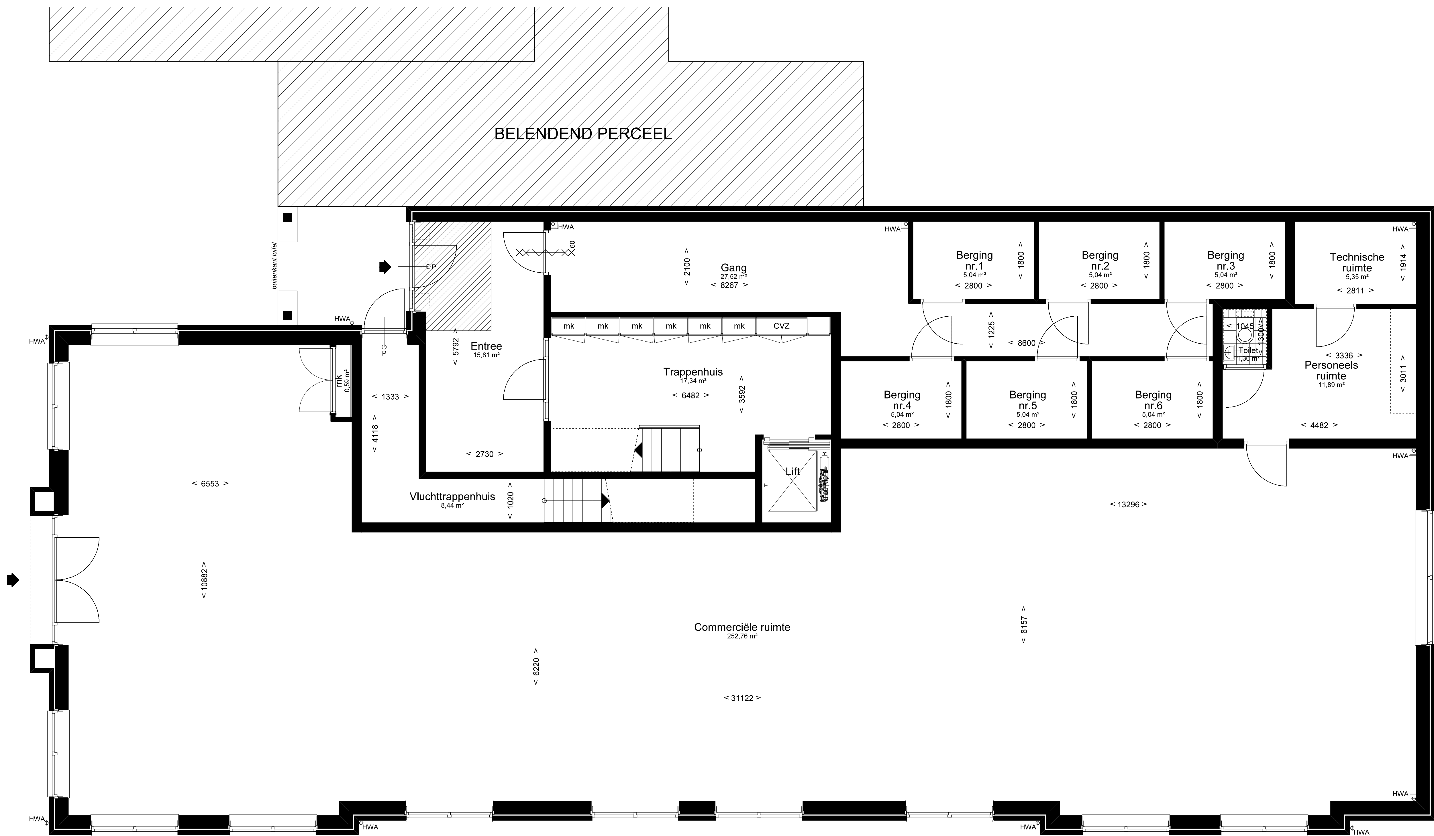
BEGANE GROND
